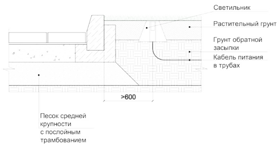
3.19 установка светильника в грунт
