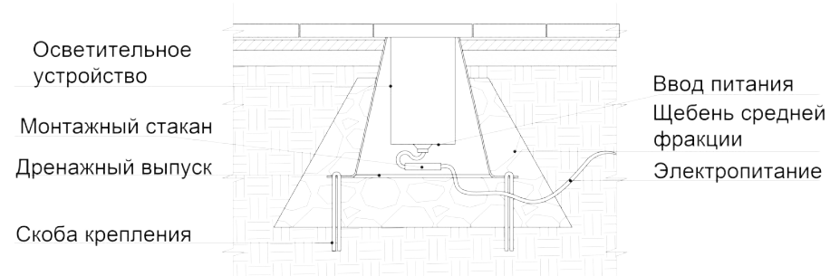
3.18 Схема установки светильника в покрытие
