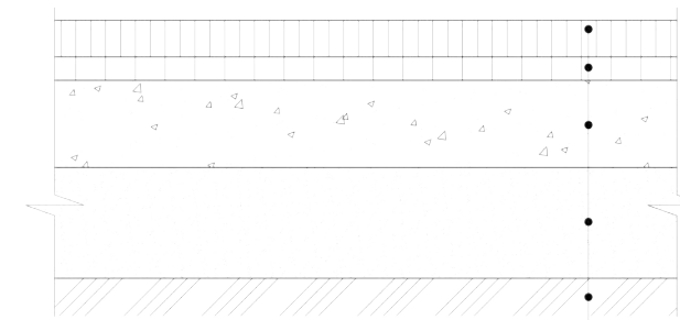
3.12 Схема устройства посевого газона
