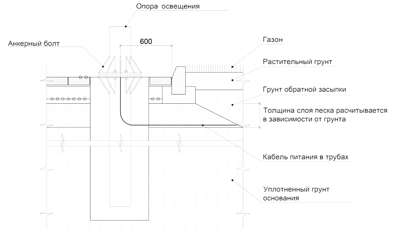
3.15 крепление опоры освещения на фланцевых закладных
