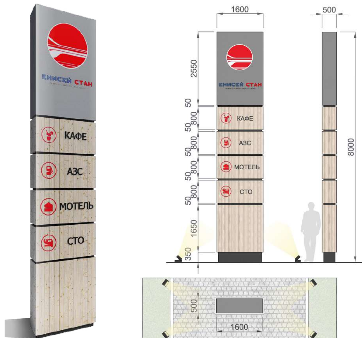
Пример стелы (конструктивное решение, вариативность заполнения модулей стелы, пиктограммы для типов ОДС)
